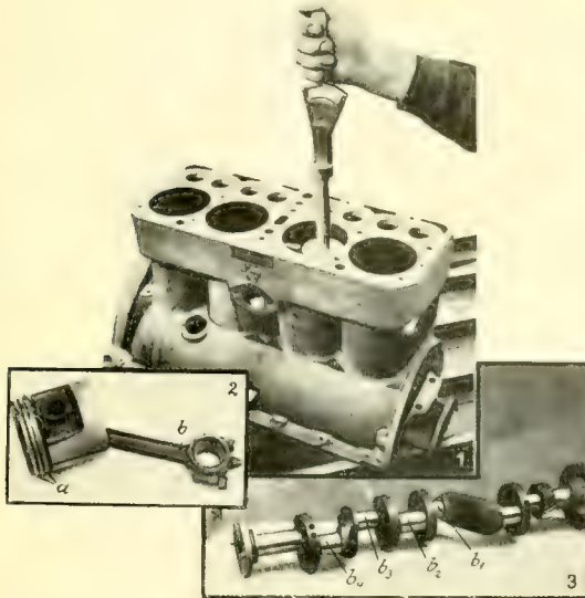
א 4-צילינדער אייטמאָביל-מאָטאָר:
